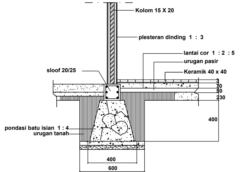
DETAIL PONDASI BATU KALI SKALA 1:20
