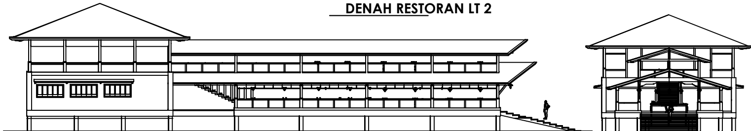
POTONGAN RESTORAN
