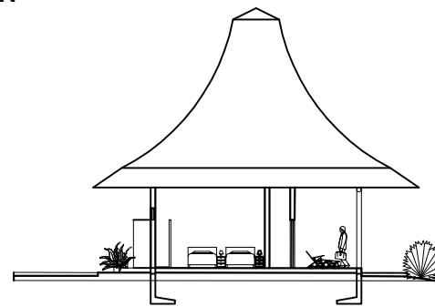
POTONGAN B-B
