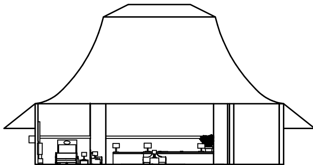
POTONGAN LOBBY
