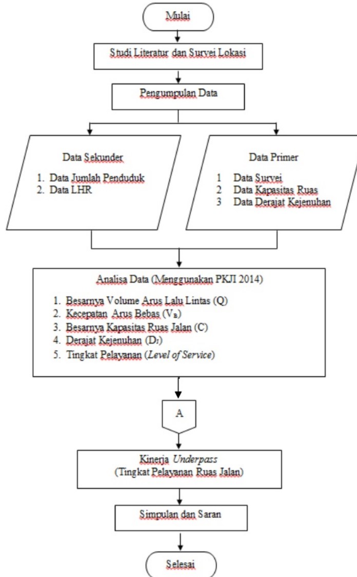
Gambar 2.1 Kerangka Penelitian
