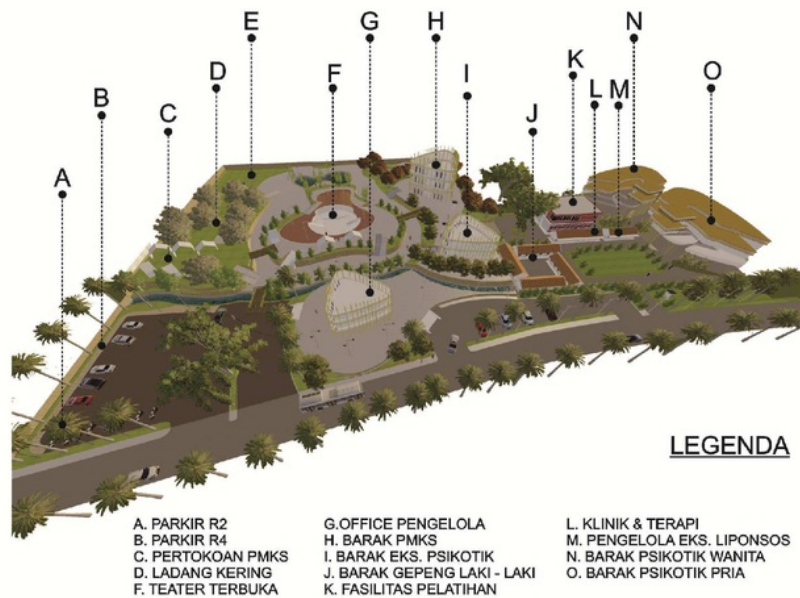
Gambar 3.6 Master Plan Pengembangan UPTD.LIPONSOS
