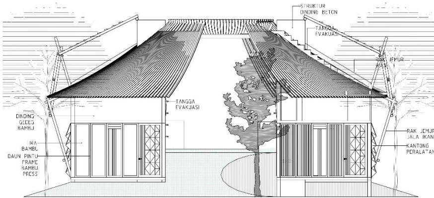
TAMPAK I
