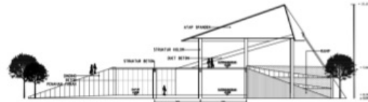
Gambar 4. Gedung Evakuasi Utama
