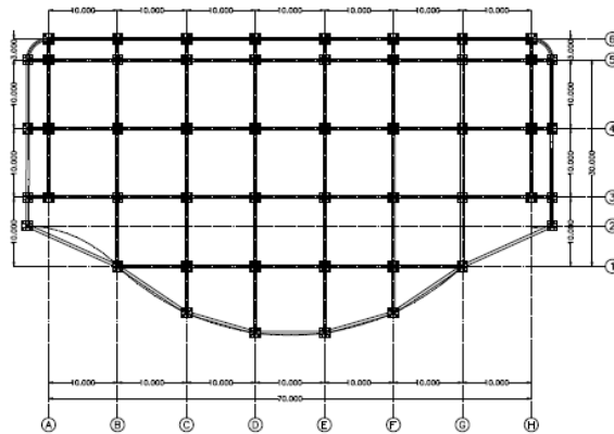
DENAH RENC. FONDASI MASSA 1 Skala 1:200
