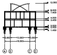
POTONGAN A-A MASSA 4 Skala 1:200
