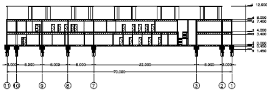
POTONGAN B-B MASSA 4 Skala 1:200
