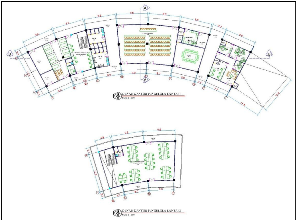
Gambar 5.18. Rencana denah kantor pengelola
