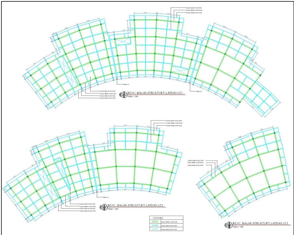
Gambar 5.31. Rencana balok struktur tempat latihan
