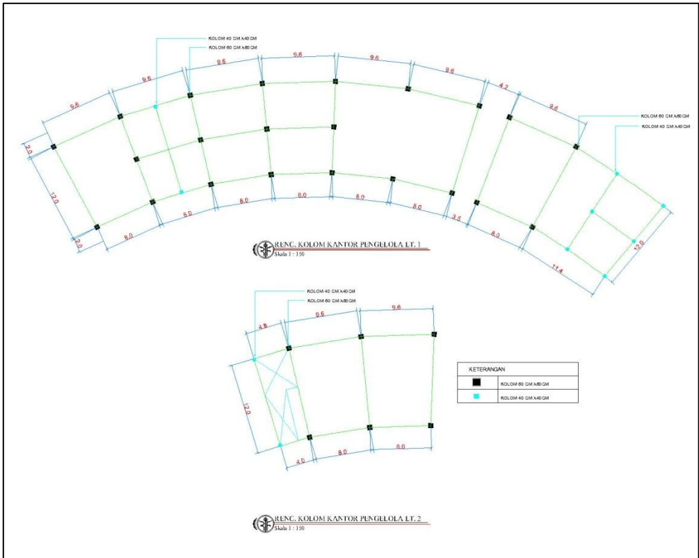
Gambar 5.23. Rencana kolom kantor pengelola
