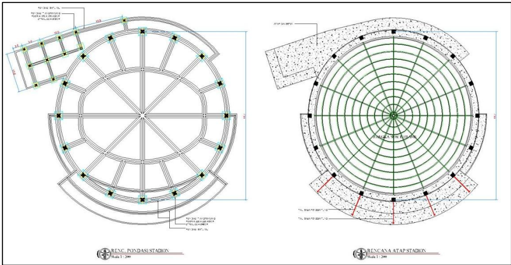
Gambar 5.15. Rencana pondasi dan atap stadion
