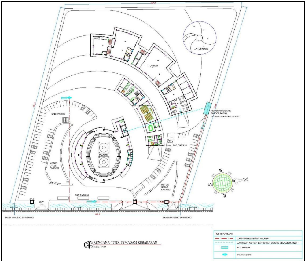
Gambar 5.10. Rencana titik pemadam kebakaran
