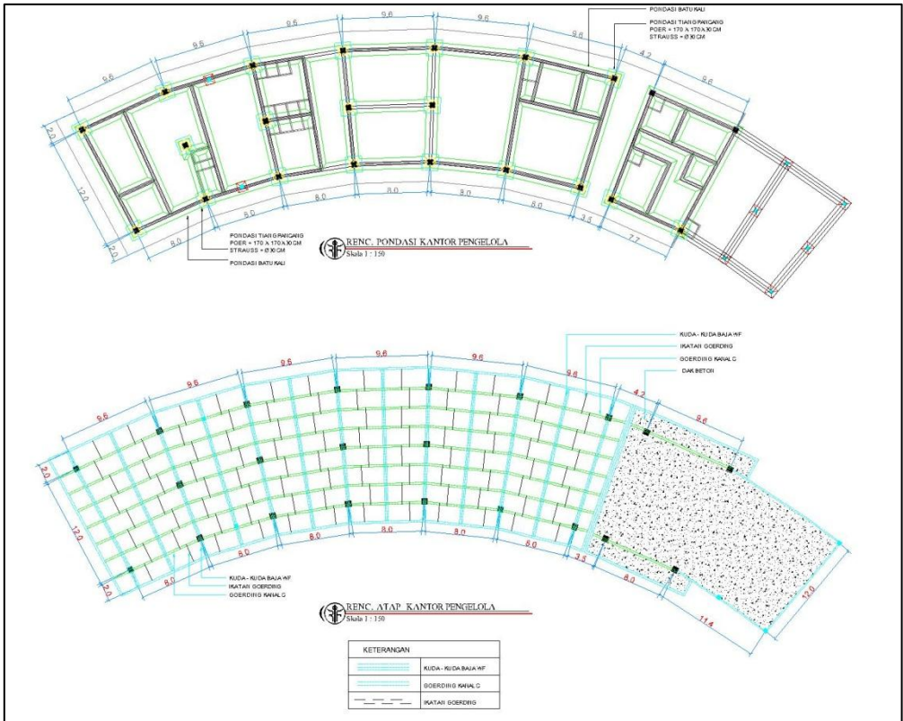
Gambar 5.22. Rencana pondasi dan atap kantor pengelola
