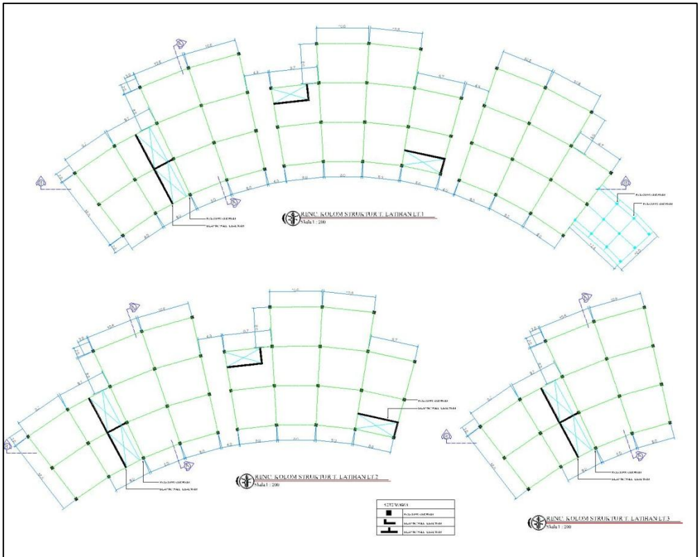
Gambar 5.30. Rencana kolom tempat latihan
