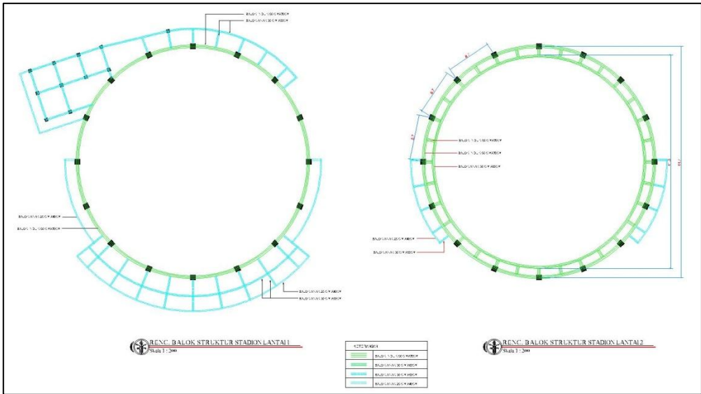
Gambar 5.17. Rencana balok struktur stadion
