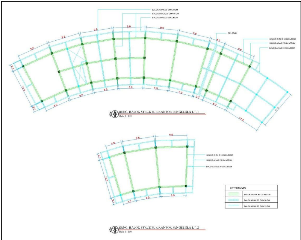
Gambar 5.24. Rencana balok struktur kantor pengelola
