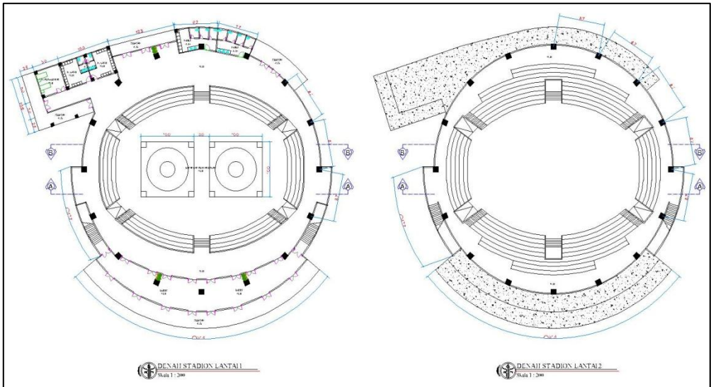
Gambar 5.11. Rencana denah stadion
