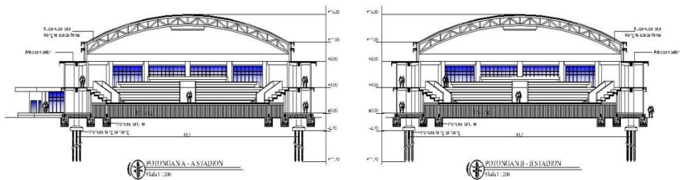
Gambar 5.14. Potongan stadion
