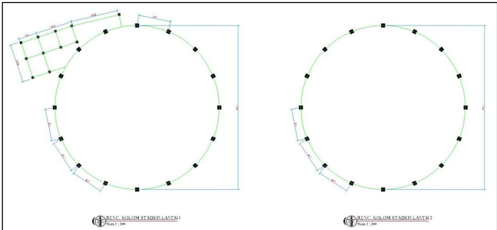
Gambar 5.16. Rencana kolom stadion
