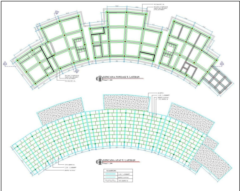
Gambar 5.29. Rencana pondasi dan atap tempat latihan
