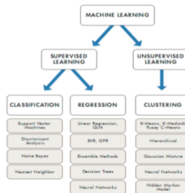
Gambar 2 Metode Pemisah Data Supervised dan Unsupervised
