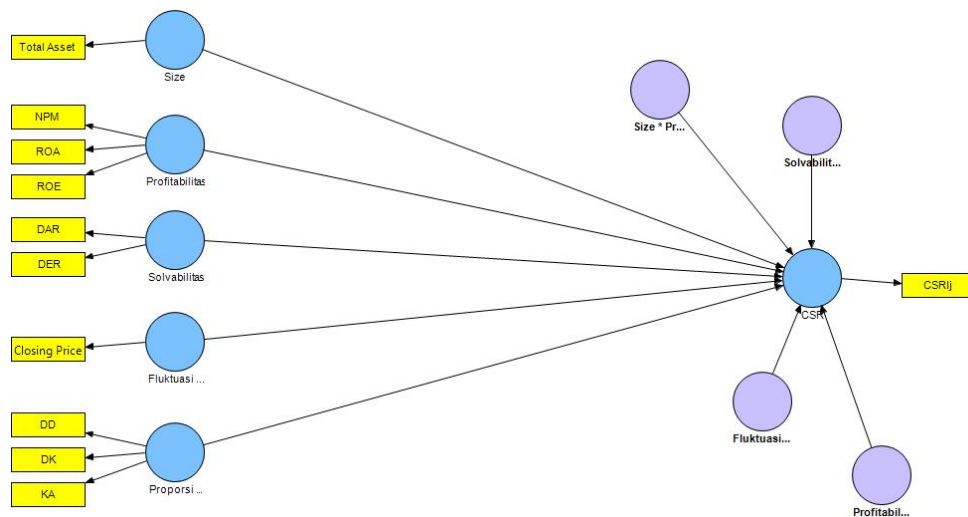
Gambar 3.1 Kerangka konseptual
