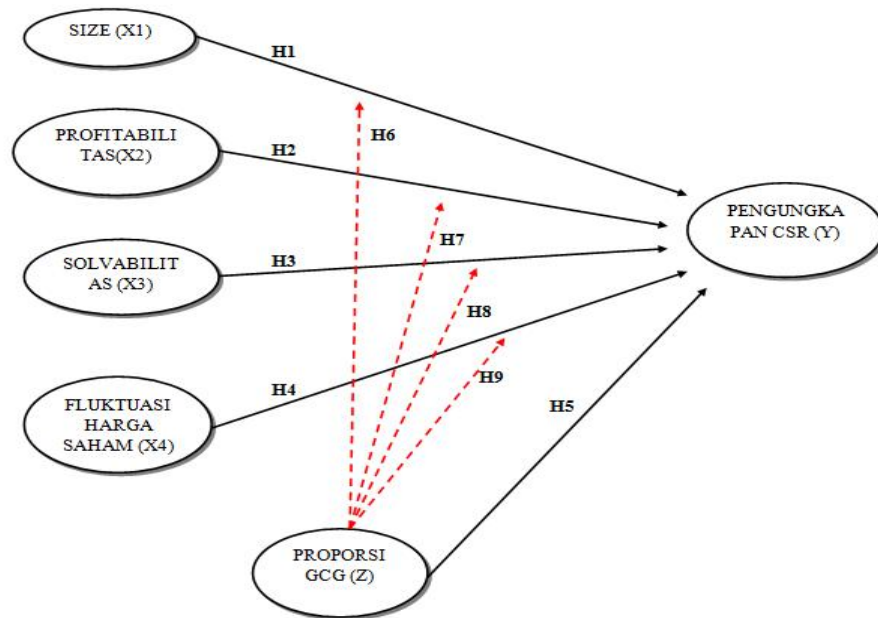
Gambar 2.1 Kerangka konseptual
