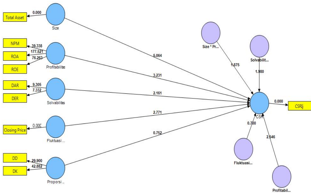
Gambar 5.3 Output Bootstarppings
