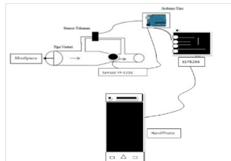
Gambar 5. Desain Alur Sistem.
