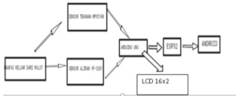
Gambar 2. Blok Diagram Alat.
