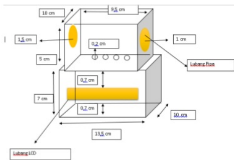
Gambar 3. Desain Tempat Alat Ukur
