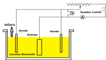
Gambar 1. Rangkaian proses elektroplating warna siver Nickel (Ni)
