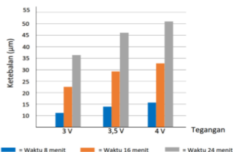
Gambar 2. Grafik hasil perhitungan ketebalan lapisan elektroplating.
