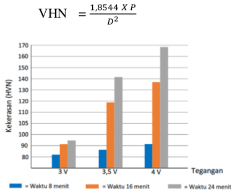
Gambar 3. grafik Perbandingan Tegangan, Waktu, dan Kekerasan mikro vickers.
