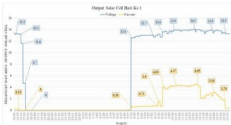
Gambar 4. Grafik pengukuran output solar cell hari ke 1
