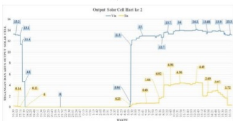
Gambar 5. Grafik pengukuran output solar cell hari ke 2
