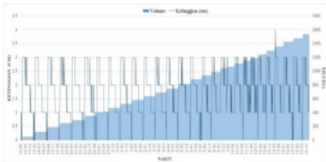
Gambar 3. Grafik pengujian sistem control hari ke 2
