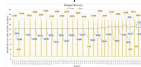
Gambar 7. Grafik pengukuran output baterai hari ke 2
