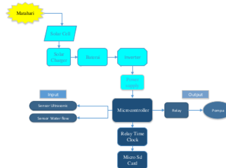
Gambar 1. Diagram blok sistem kerja alat
