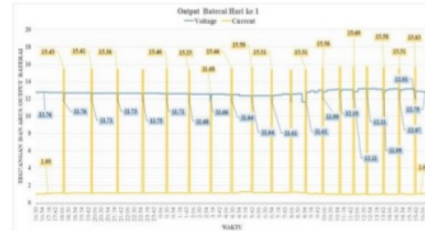
Gambar 6. Grafik pengukuran output baterai hari ke 1
