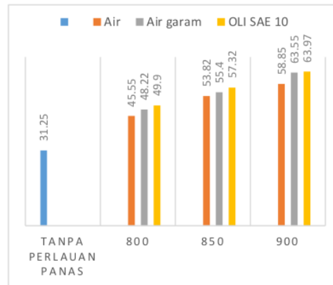
Gambar 1. rekapitulasi hasil uji kekerasan
