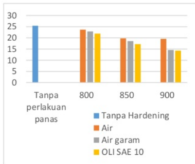
gambar 3. grafik energi impact
