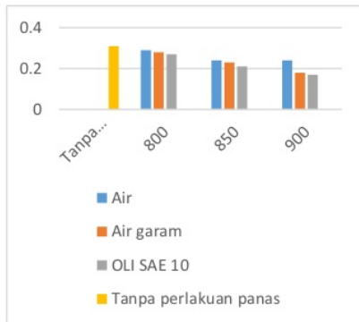
Gambar 2. grafik harga impact
