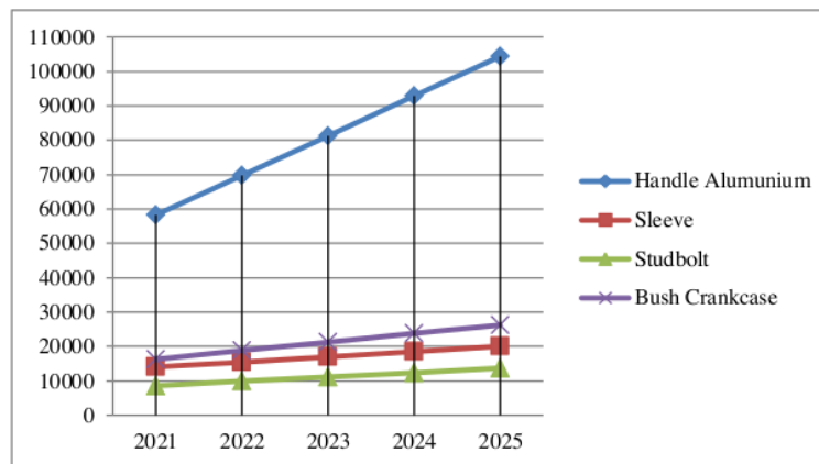
Gambar 4.1 Diagram Peramalan 5 tahun ke depan
