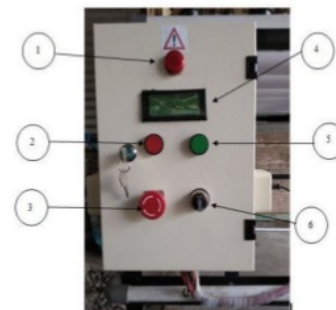
Gambar 3.6 panel box kontrol luar
