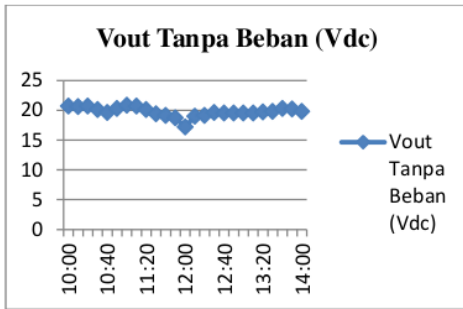
Gambar 4. Grafik Pengukuran Tegangan Tanpa Beban
