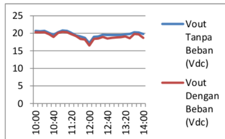
Gambar 8. Grafik Pengukuran Tegangan Tanpa Beban & Dengan Beban
