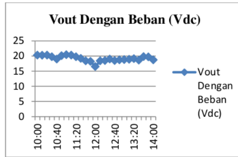
Gambar 6. Grafik Pengukuran Tegangan Dengan Beban
