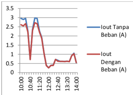
Gambar 9. Grafik Pengukuran Arus Tanpa Beban & Dengan Beban
