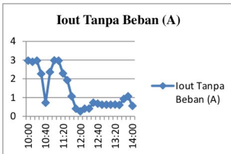
Gambar 5. Grafik Pengukuran Arus Tanpa Beban
