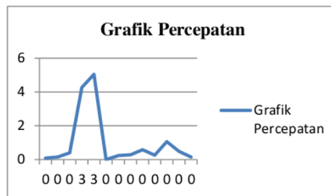
Gambar 12. Grafik Percepatan Getaran Kecil & Jarak 30 CM
