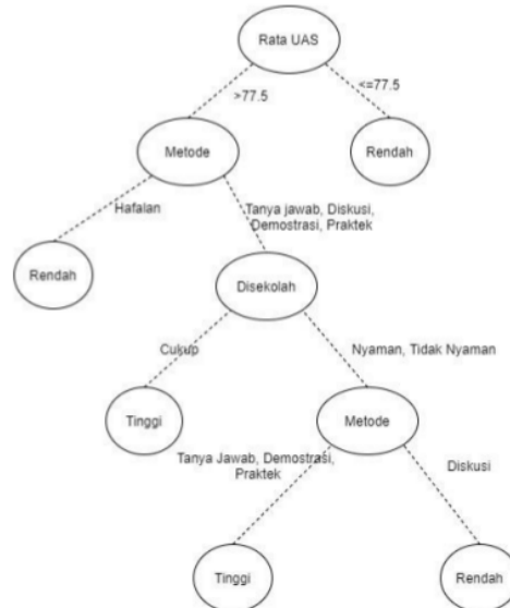
Gambar 8 Pohon Keputusan
