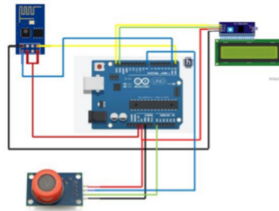
Gambar 3. Rancangan Komponen Elektronika
