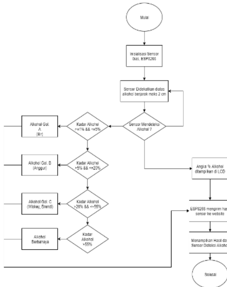
Gambar 2. Flowchart Perangkat Keras
