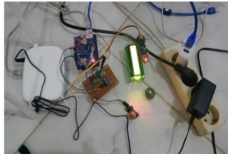
Gambar 5. Rangkaian Keseluruhan Alat
