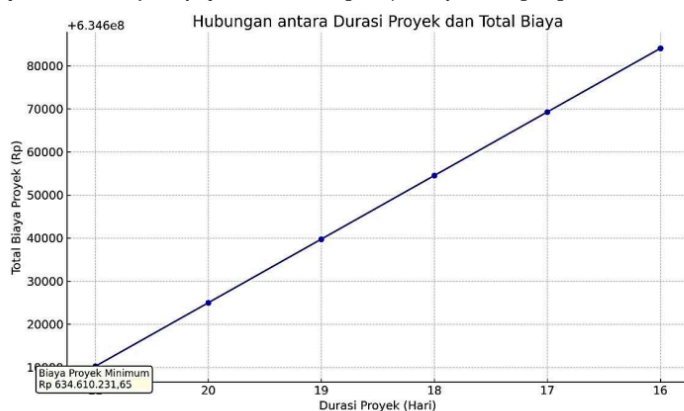
Gambar 2. Grafik Hubungan Antara Durasi Proyek Dan Total Biaya
