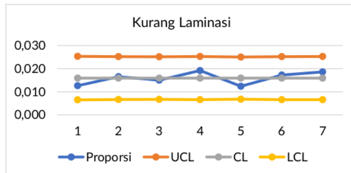
Gambar 3. 5 Grafik Peta Kendali Jenis Cacat Kuarng Laminasi
