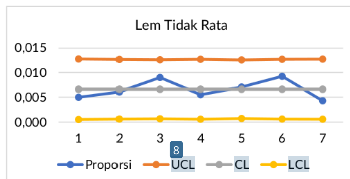
Gambar 3. 6 Grafik Peta Kendali Jenis Cacat Lem Tidak rata
