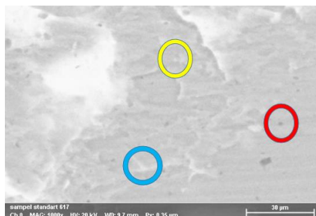
Gambar 12. Analisa Spesimen K1
