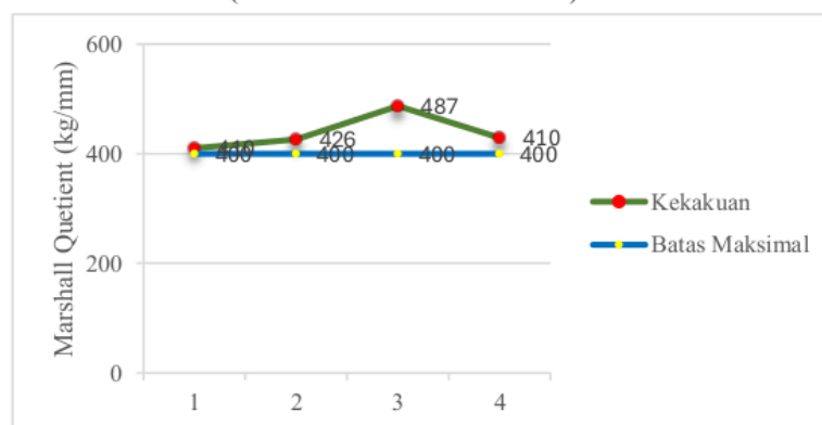
Grafik 2. Uji Marshall pada kondisi KAO
