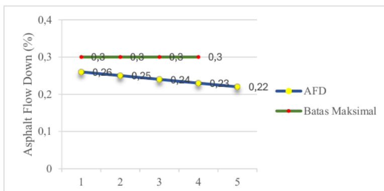
Grafik 1. Uji Asphalt Flow Down
