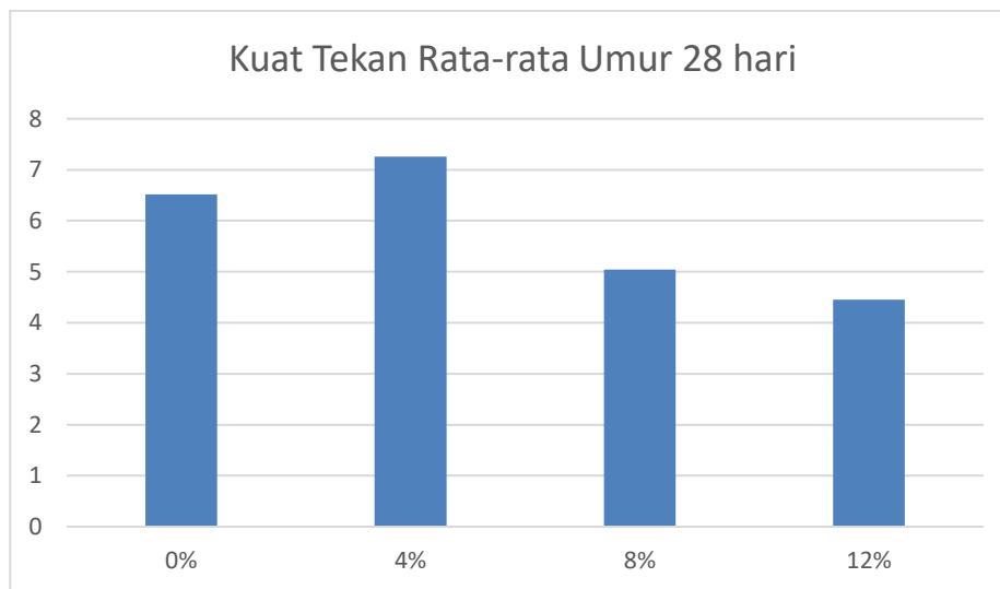
Gambar 4 Grafik Kuat Tekan Rata-rata Umur 28 hari
