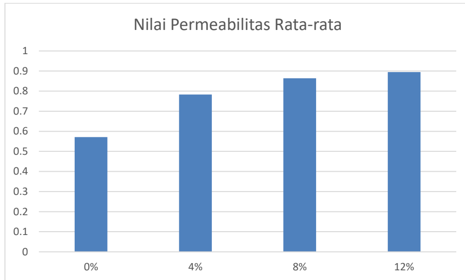
Gambar 6 Grafik Permeabilitas Rata-rata
