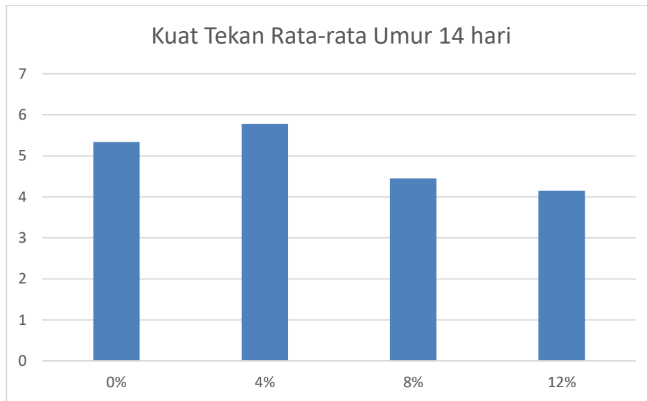
Gambar 3 Grafik Kuat Tekan Rata-rata Umur 14 hari
