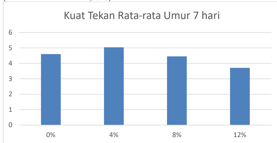
Gambar 2 Grafik Kuat Tekan Rata-rata Umur 7 hari
