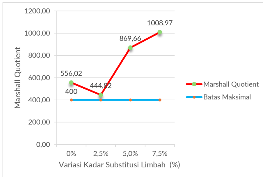
Gambar 3. Grafik Hubungan Kadar PET terhadap Marshall Quotient
