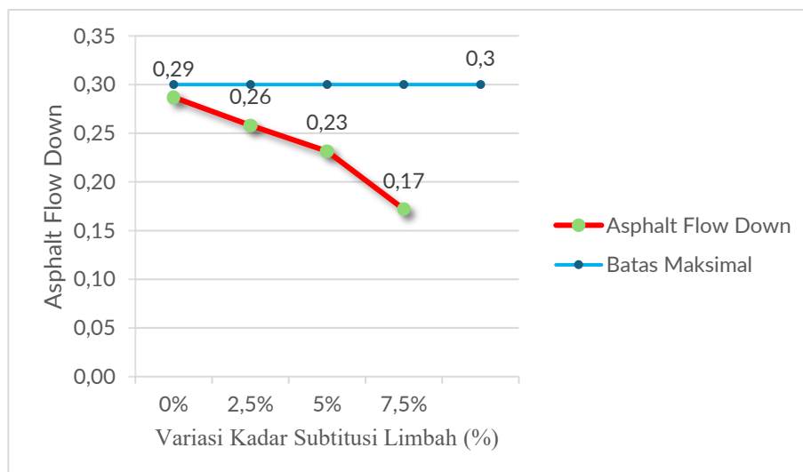
Gambar 5. Grafik Hubungan Kadar PET terhadap Asphalt Flow Down
