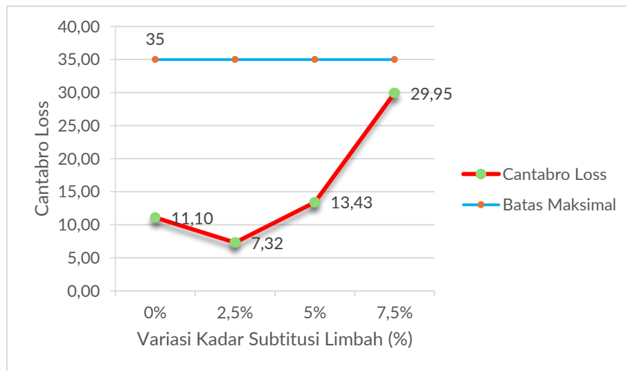
Gambar 4. Grafik Hubungan Kadar PET terhadap Cantabro Loss
