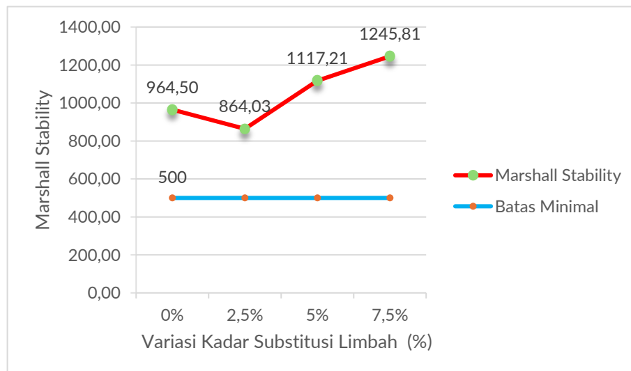
Gambar 1. Grafik Hubungan Kadar PET terhadap Marshall Stability
