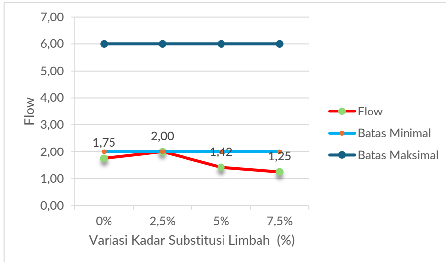
Gambar 2. Grafik Hubungan Kadar PET terhadap Nilai Flow
