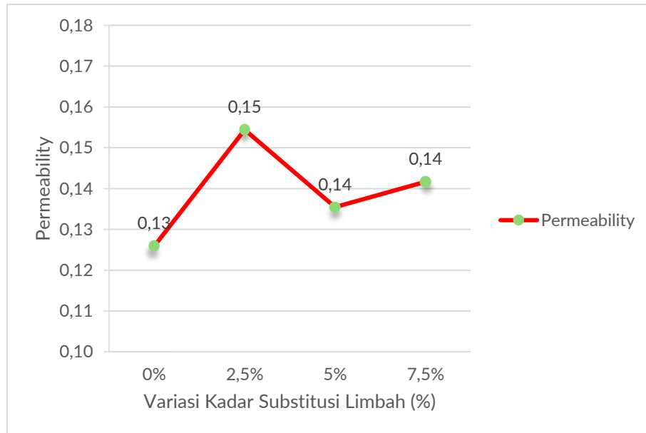
Gambar 6. Grafik Hubungan Kadar PET terhadap Permeability
