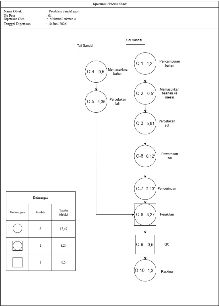
Lampiran 2 OPC Produksi Sandal
