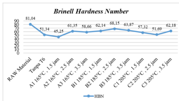
Gambar 3. Grafik Rekapitulasi Nilai Kekerasan
