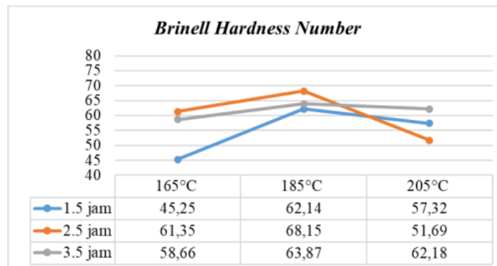
Gambar 2. Pengaruh temperatur pada setiap waktu aging
