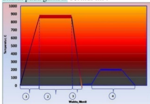
Gambar 1 siklus heat treatment pada baja
