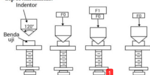
Gambar 3 Proses pengujian kekerasan rockwell
