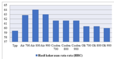
Grafik 1. Data hasil uji kekerasan
