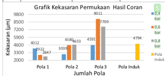
Gambar 7 Grafik Kekasaran Permukaan
