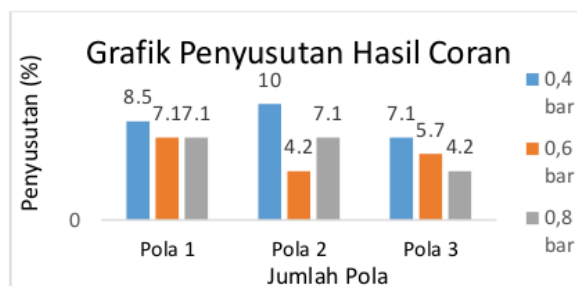
Gambar 6 Grafik Penyusutan
