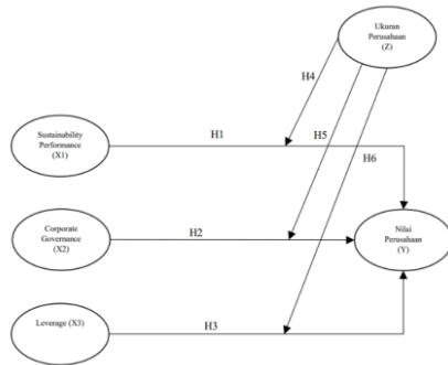
Gambar 1. Kerangka Konseptual
