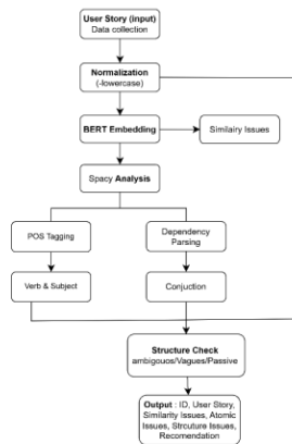
Gambar 1. Alur Pra-pemrosesan dan Analisis Sintaksis User Story
