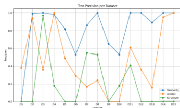
Gambar 4. Grafik Tren Precision per Dataset
