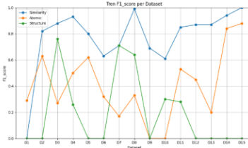
Gambar 6. Grafik Tren F1-Score per Dataset
