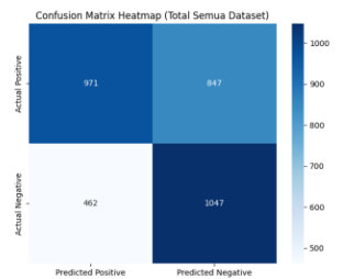
Gambar 3. Distribusi Klasifikasi Berdasarkan Confusion Matrix
