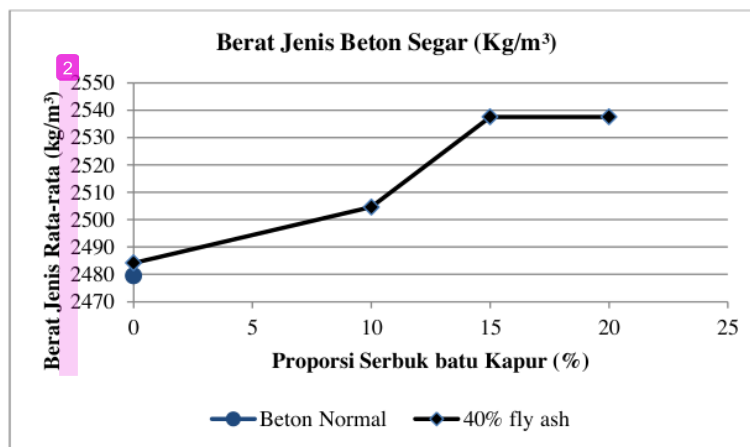
2 Gambar 4 Grafik Analisa Hasil Nilai Berat Jenis Beton Segar
