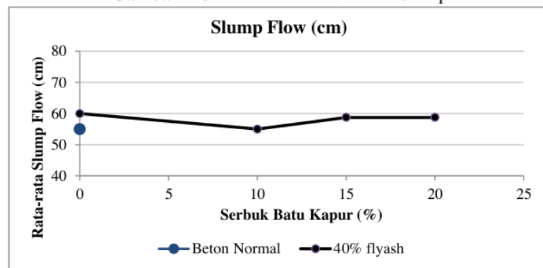
Gambar 3 Grafik Analisa Hasil Nilai Flow
