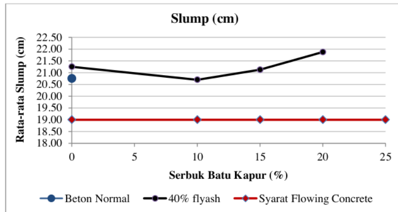
Gambar 2 Grafik Analisa Hasil Nilai Slump
