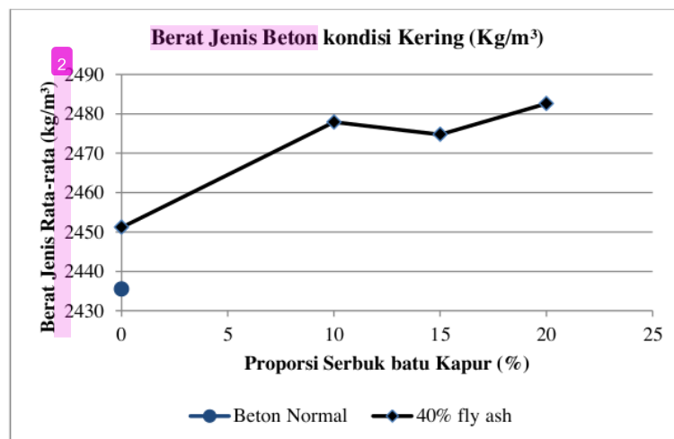
2 Gambar 5 Grafik Analisa Hasil Nilai Berat Jenis Beton kondisi Kering
