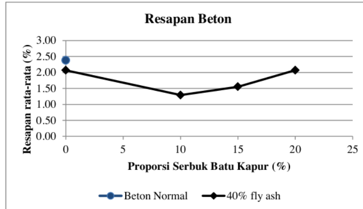
Gambar 6 Grafik Analisa Hasil Nilai Resapan Beton
