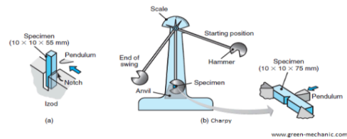
Gambar 1 Pengujian impact
