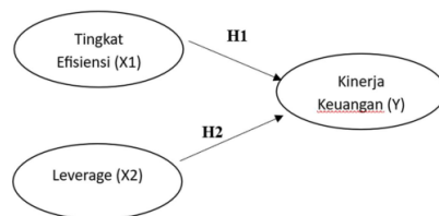
Gambar 1. Kerangka Konseptual
