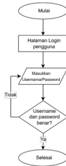
Gambar 2 Flowchart Sistem Login
