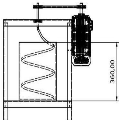
Gambar Kerangka Pengaduk Adonan Tampak Samping
