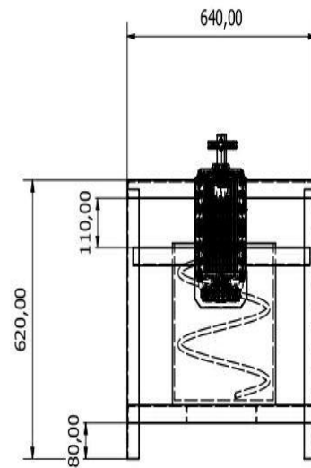
Gambar Kerangka Pengaduk Adonan Tampak Depan
