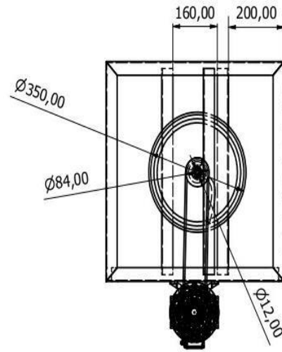
Gambar Kerangka Pengaduk Adonan Tampak Atas
