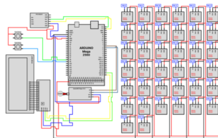
Gambar. 3 Desain Rancangan
