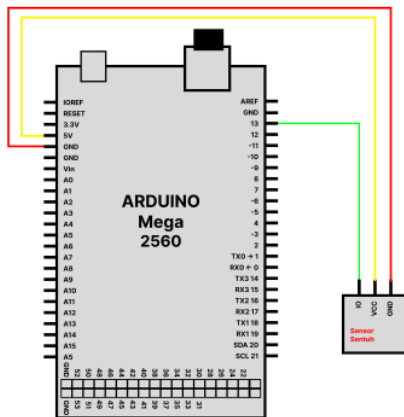
Gambar. 4 Rangkaian sensor sentuh
