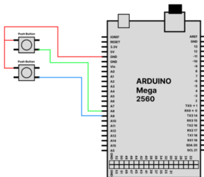
Gambar. 5 Rangkaian tombol tekan
