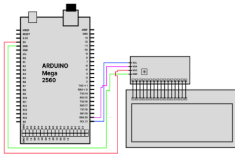
Gambar. 8 Rangkaian LCD I2C 20x4
