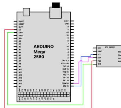
Gambar. 7 Rangkaian Modul RTC DS3231
