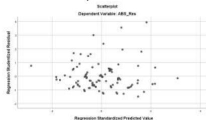
Gambar 1 Uji Heteroskedastisitas
