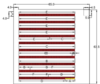
Gambar 2 Layout Usulan Gudang Bahan Baku
