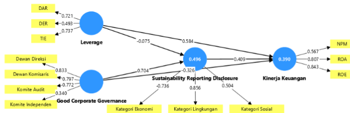
Gambar 1. Diagram jalur dan nilai loading factor sebelum eliminasi indikator
