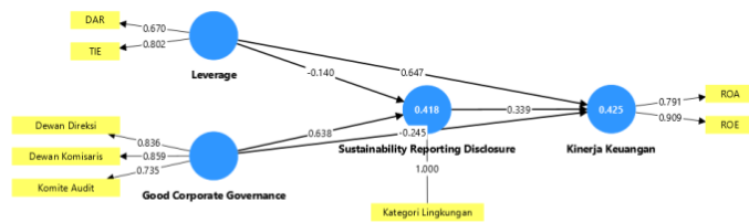
24 Gambar 3. Diagram jalur dan nilai loading factor setelah eliminasi indikator
