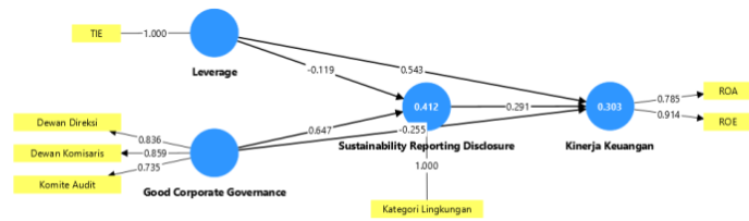
Gambar 5. Diagram jalur dan nilai loading factor setelah eliminasi indikator kedua
