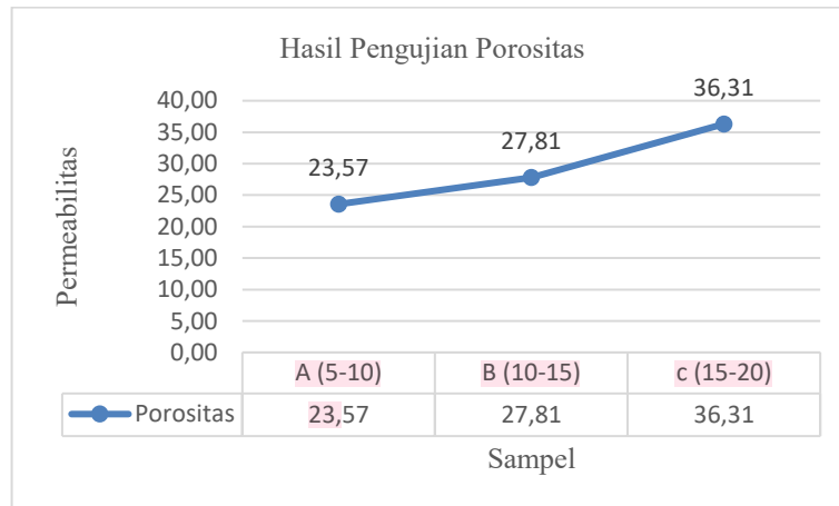
Gambar 3 Grafik Hasil Pengujian Porositas
