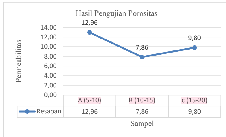
Gambar 4 Grafik Hasil Pengujian Porositas
