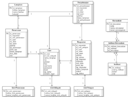
Gambar 4. Relasi Tabel
