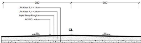
Gambar 1. Potongan Perkerasan Lentur Ruas Jalan Serah - Tebuwung
