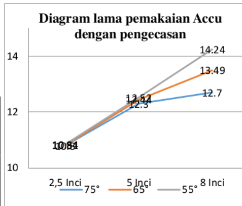
Gambar 1. Diagram Pemakaian Accu Berdasarkan dengan pengujian dan analisis data yang telah dilakukan, maka dapat disimpulkan :
