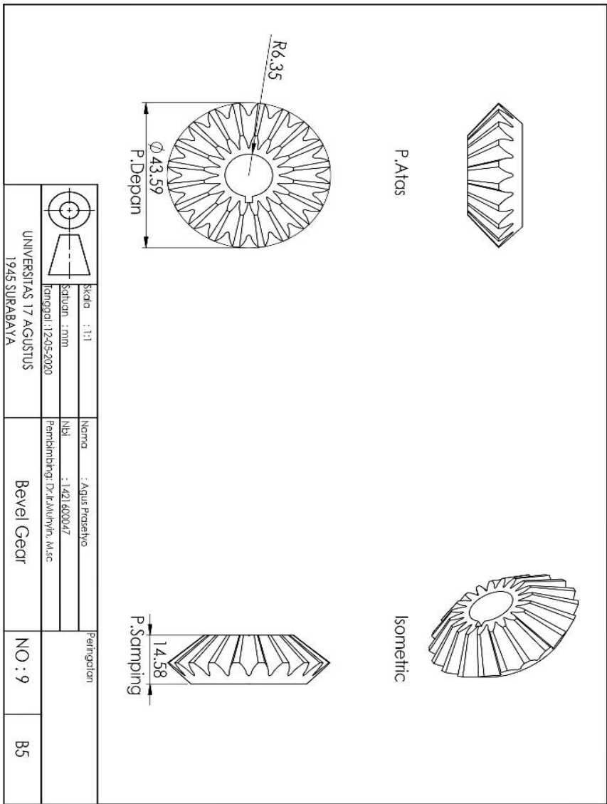
Gambar teknik bevel gear.
