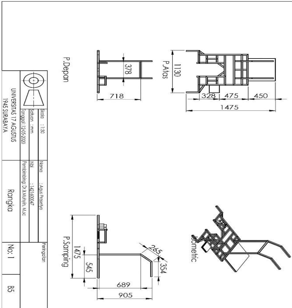
Gambar teknik kerangka mesin.
