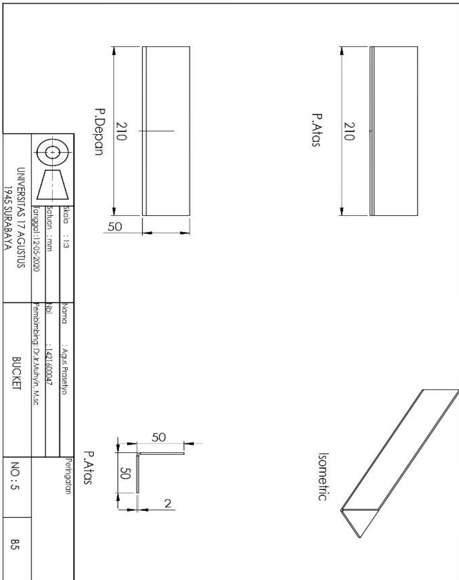
Gambar teknik bucket elevator.
