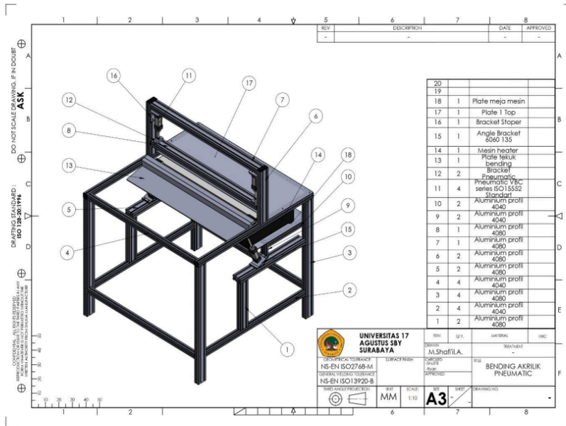
Gambar 2 Detail pada mesin bending
