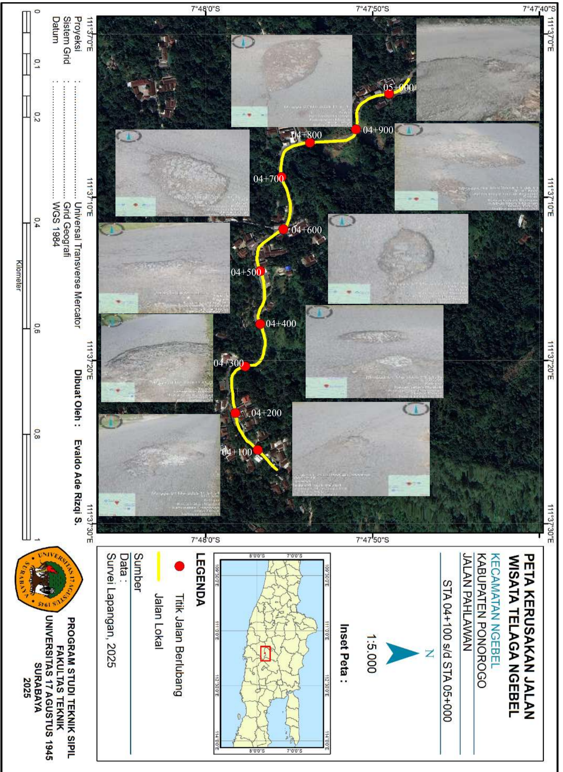
Gambar L. 5 Peta Kerusakan Jalan STA 04+100 Sampai 05+000
