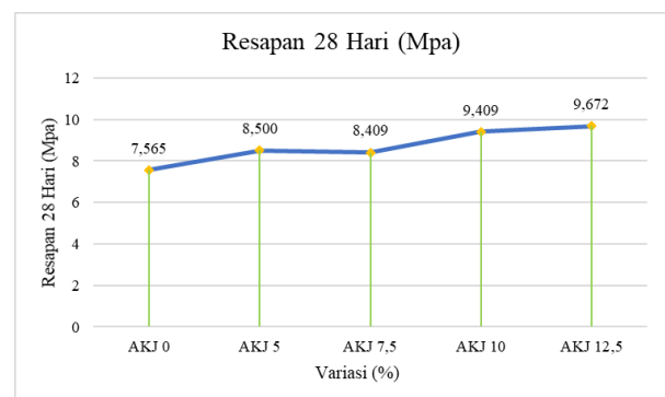
Gambar 4. Grafik Resapan Air Mortar
