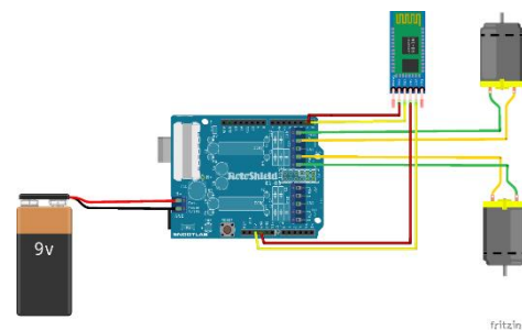
Gambar 3. Rangkaian Mobile Robot
