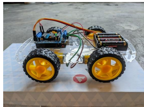
Gambar 7. Bagian Mobile Robot
