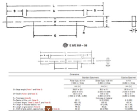
Gambar 2. Spesimen uji sesuai standar ASTM E8
