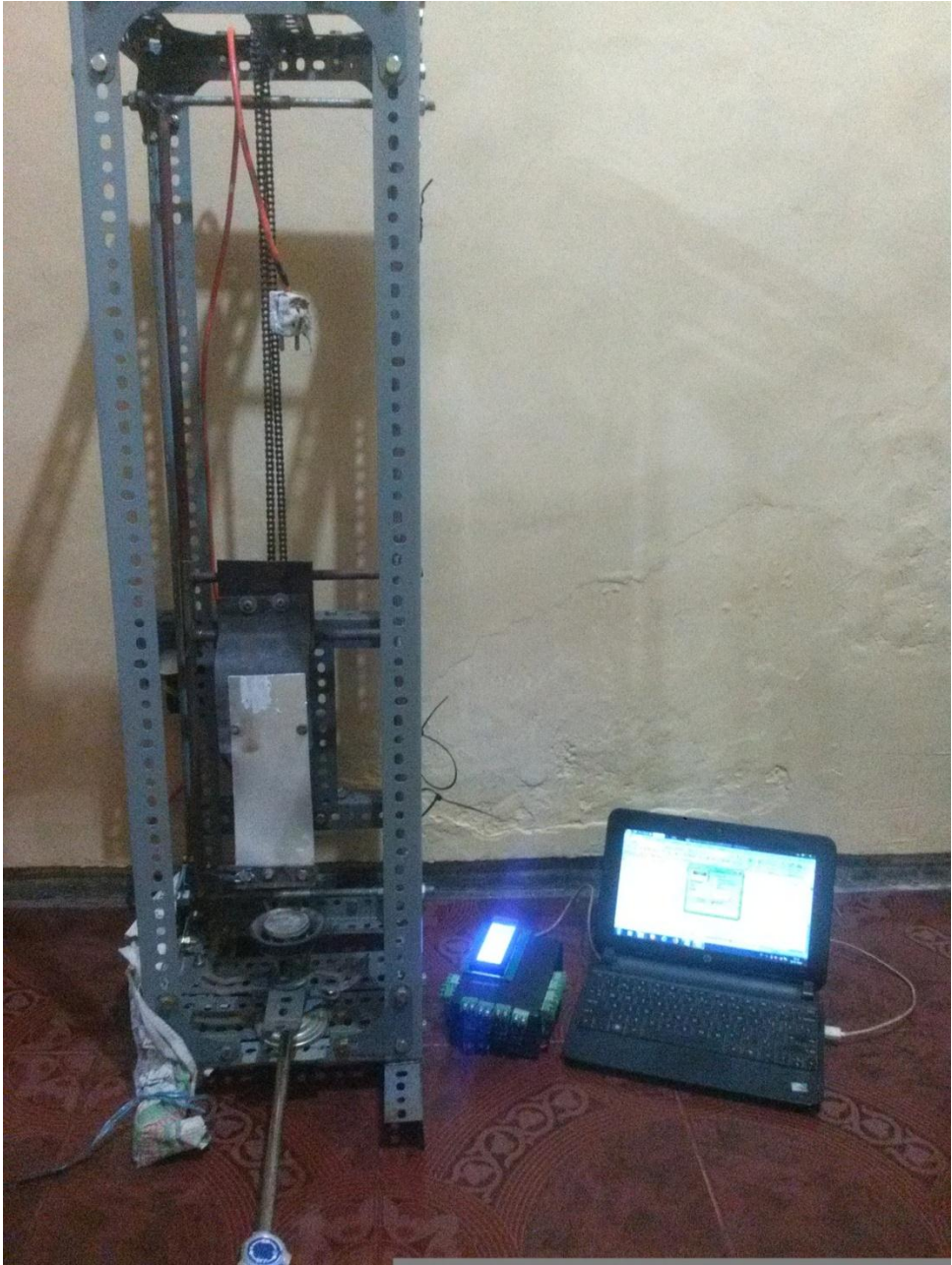
Instalasi percobaan
